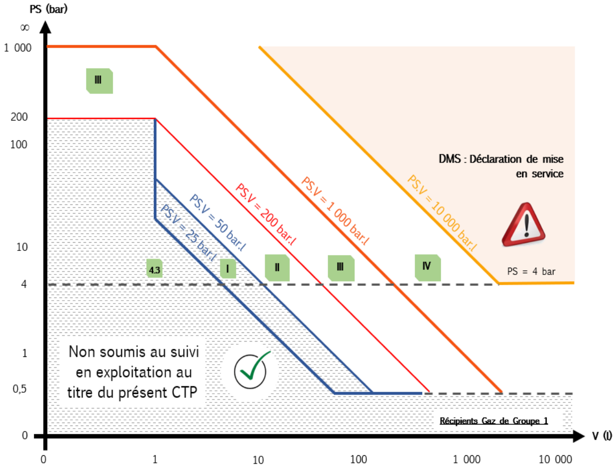
Extrait du Tableau 1 Annexe II de la Directive 2014/68/UE Réceptifs visés à l'article 4, paragraphe I point a), i) tiret un
