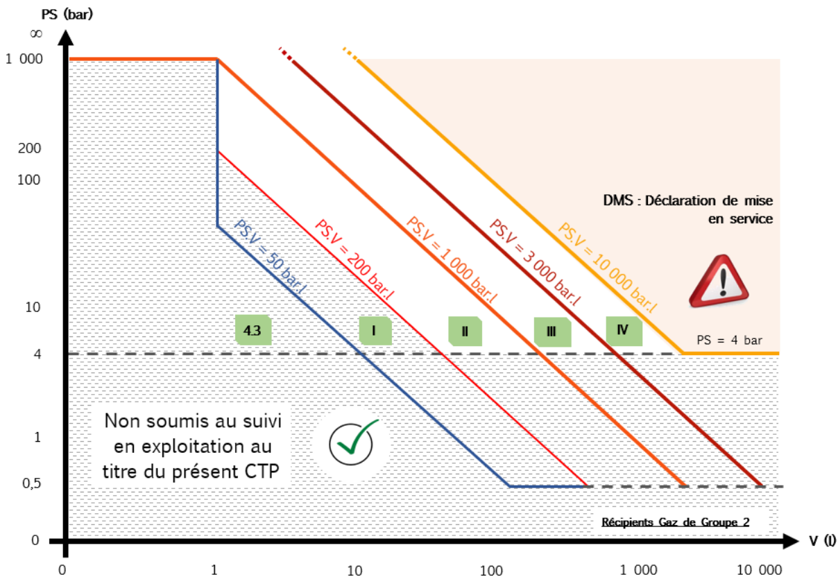
Extrait du Tableau 2 Annexe II de la Directive 2014/68/UE Réceptifs visés à l'article 4, paragraphe I point a), i) tiret deux
